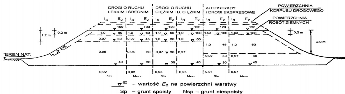
Rysunek 3 - Wartości wymagane w nasypach: wskaźnika zagęszczenia I_s i wtórnego modułu odkształcenia E_2 , megapaskali
