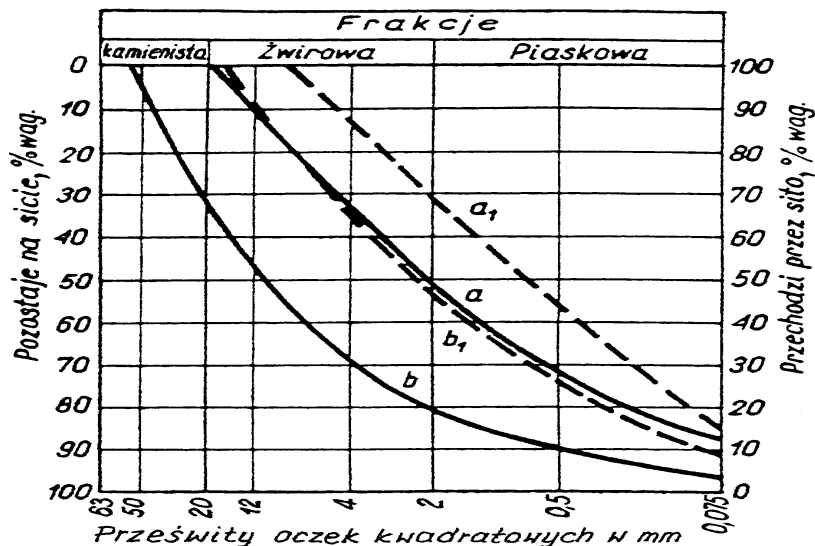
Rysunek 1. Obszar uziarnienia optymalnych mieszanek żwirowych
